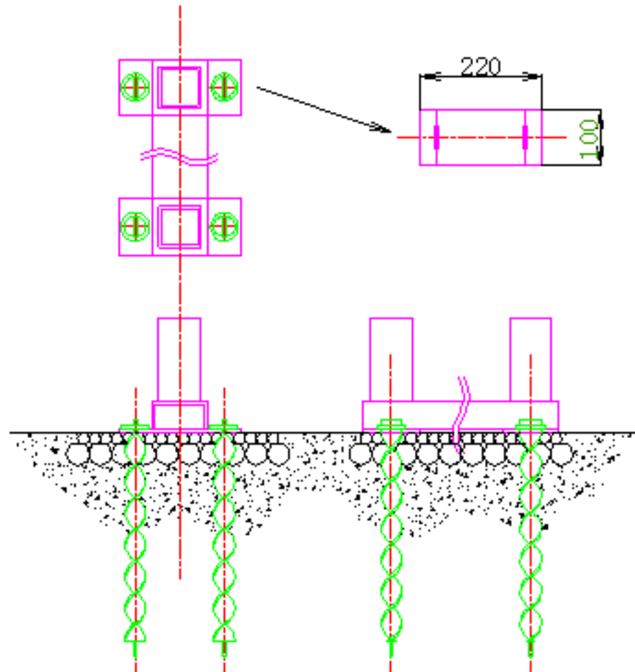
参考使用杭 6*38*400
