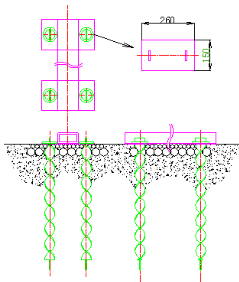
参考使用杭 6*50*600
